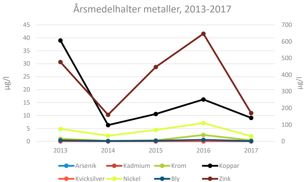
Figur 5 Årsmedelhalter för vissa metaller under de fem senaste åren. Observera att Zn redovisas på sekundäraxeln.
