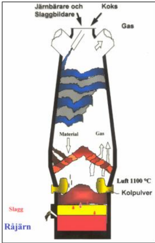
Figur 1. Masugnsprocessen.
